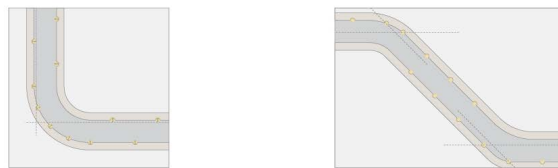
Disposición de luminarias en tramos curvos
